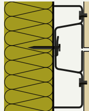
PlankClip op hout (met isolatie)
