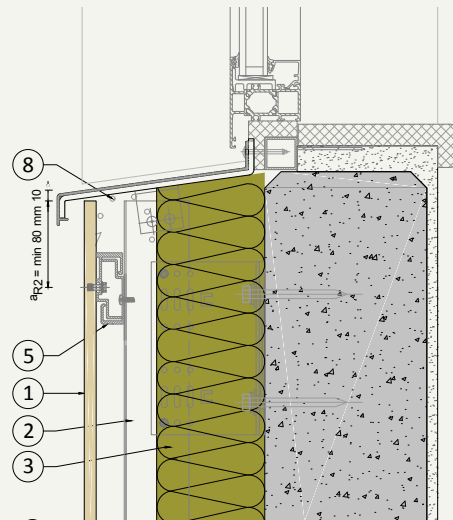
V.04 Vensterbank aansluiting
